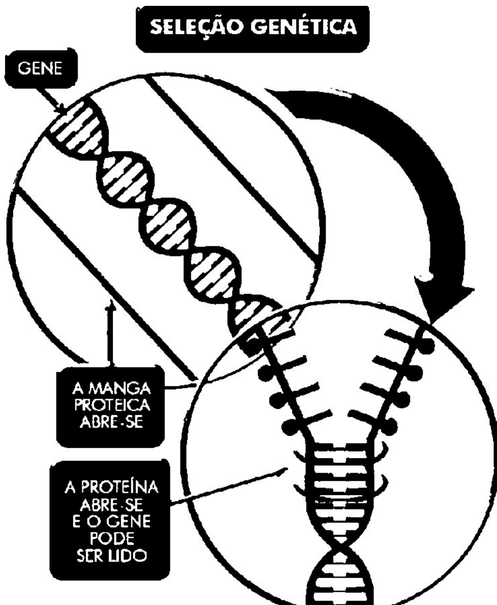
A Figura 4.2B ilustra a forma como a manga proteica em torno da sequência genética do ADN se abre para que uma outra proteína chamada proteína regulatória possa abrir e ler o gene numa localização específica.
